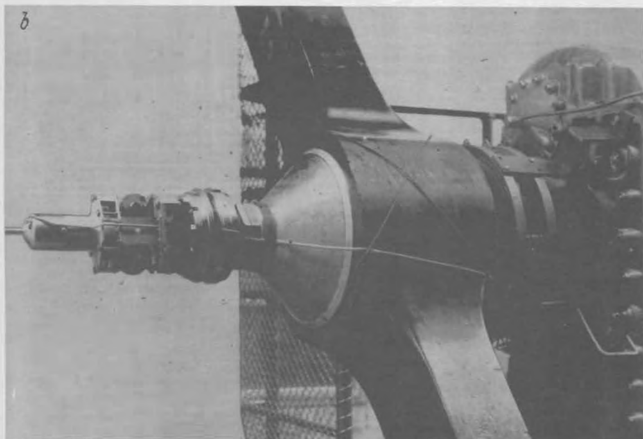
Abb. 3 DVL-Drehmomentschreiber am Jumo 205; a) Einzelteile b) Gesamtansicht am Motor.
