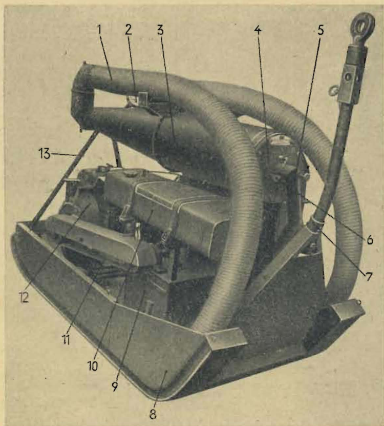
Bild 1 Vorwärmgerät, Vorderansicht
