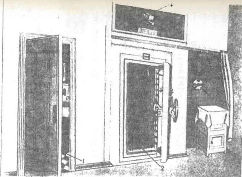
Рис. 9. Внешний вид части палаты биотрона: 1 — санузел; 2 — входной шлюз; 3 — почтовый шлюз; 4 — поворотная телевизионная головка.
