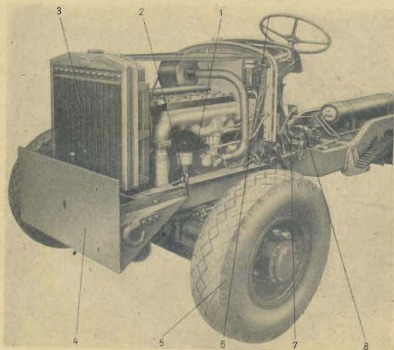
Bild 2 Vorderansicht des Kraftfahrzeuges
