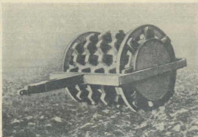
Abb. 51. Schaffuwalze der Fa. Menck & Hambrock.
