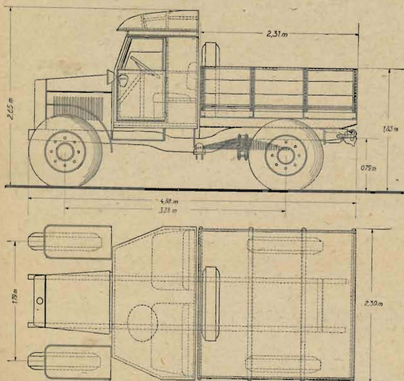
Bild 1 Radschlepper „Laffly R 35“
