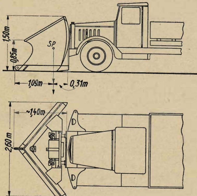
Bild 29 Vorbauschneepflug „EPK 2 Radstadt“ (Bauart Scheid)
