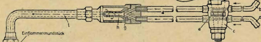
B Niederdruck-(Saug-) brenner (für Azetylen)
