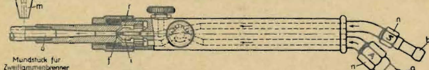
C Hochdruck-(Gleichdruck-) brenner (für Azetylen)
