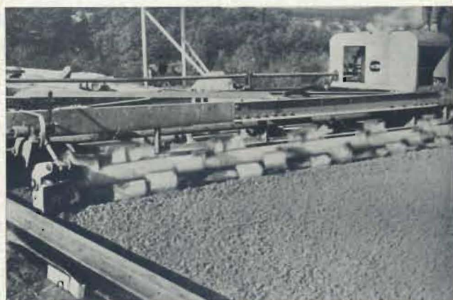
Bild 9: Verteilter Beton vor dem Straßenfertiger.
