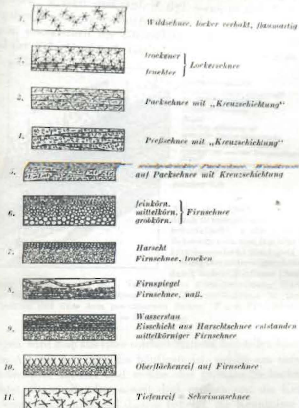
Abb. 70. Schematische zeichnerische Darstellung der Schneearten zur Verwendung bei der Wiedergabe von Schneeprofilen (Schichtenfolgen).
