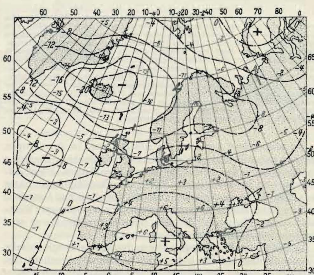
Abb. 1g. 850 mb Vergleich mit der weiteren mittleren Änderung bis 21. 1., 15 Uhr
