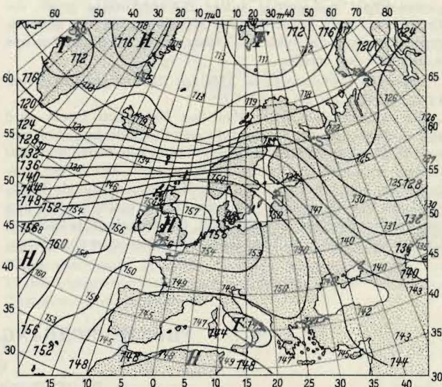
Abb. 1f. 850 mb Vergleich mit der erweiterten Vorhersage 17. 1., 15 Uhr bis 20. 1., 15 Uhr
