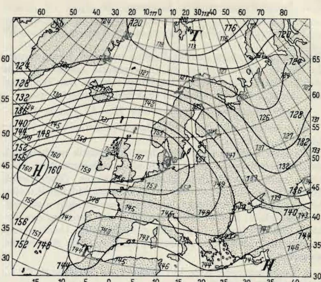
Abb. 1 e. 850 mb Vergleich mit der Vorhersage 17. 1., 3 Uhr bis 19. 1., 3 Uhr
