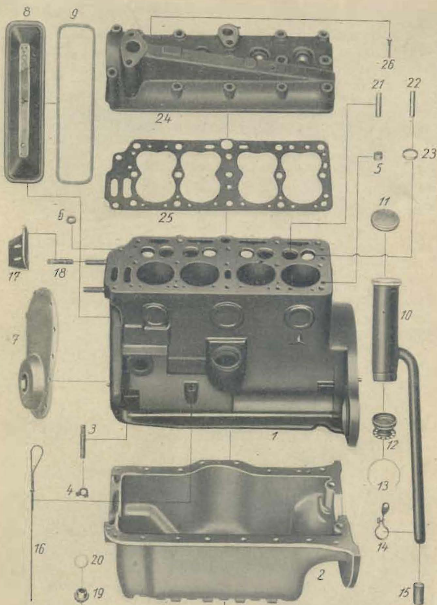
Tafel 1. Gruppe M: a) Motor Kurbelgehäuse, Zylinderkopf
