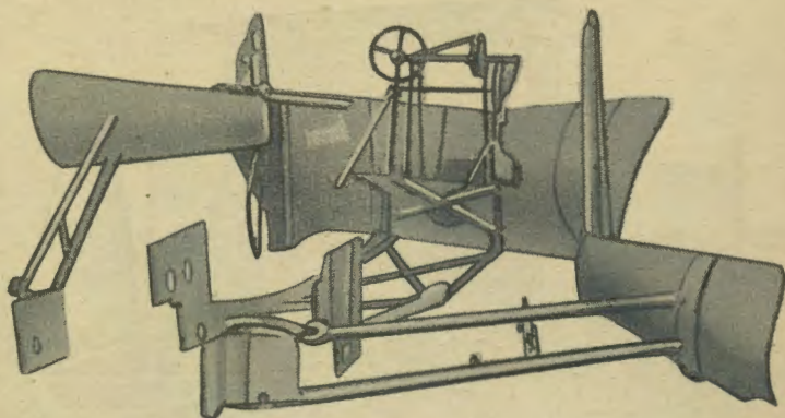
Abb. 70 a: Einzelheiten des kombinierten Schneeräumers Wausau. (Rückansicht.)
