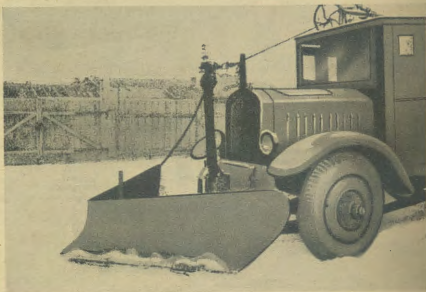
Abb. 71; Keilflug sowjetischer Fabrikation, hergestellt im Werk Onega an einem 5-t-Lkw. des Werkes Jaroslaw, Type J-5.
