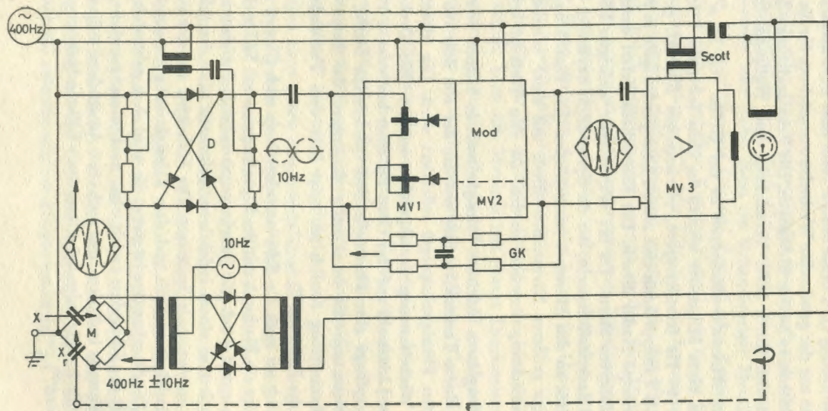
Bild 2.20. Kapazitive Aufnehmer mit Trägerfrequenz-Nullstrom
